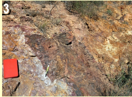
Antiguo filón sulfurado completamente transformado en goethita y óxidos de Mn. En el contacto la dacita porfírica está fuertemente alterada a caolinita.
